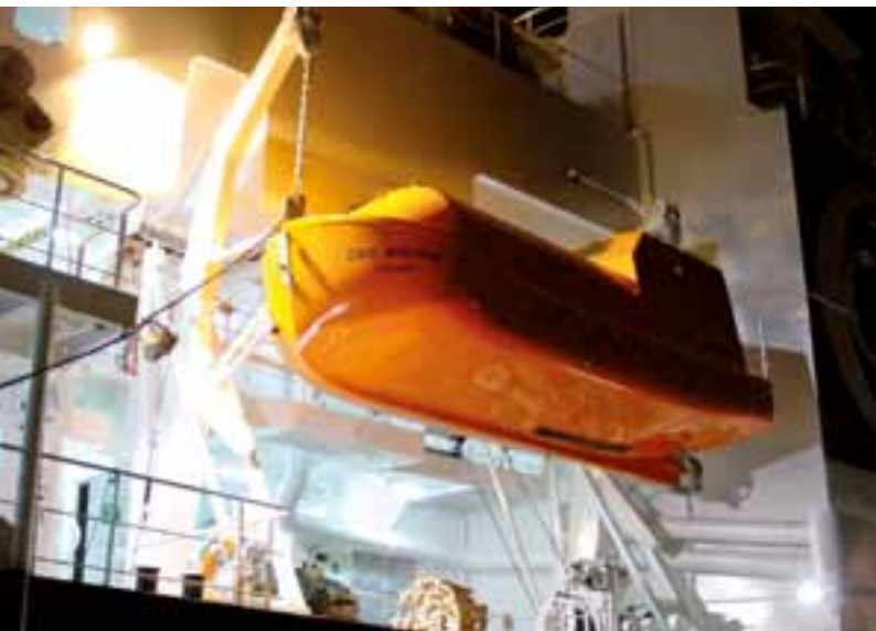
Fassmer Pivot Davit | FPD
